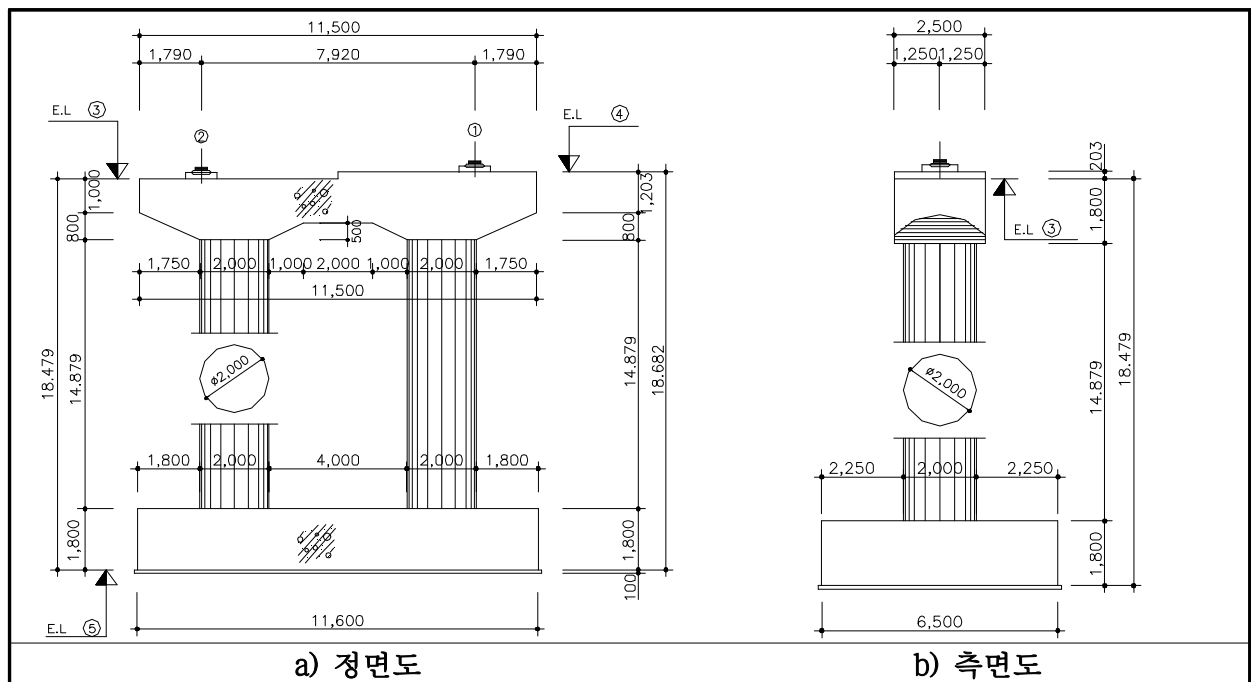
【그림 5.5】 해석단면
